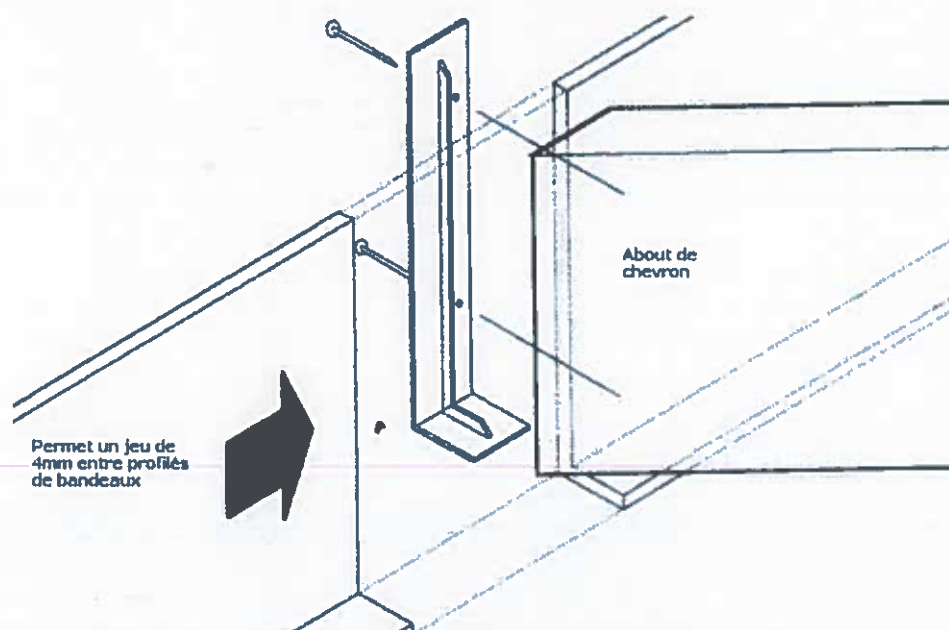
Figure 17 – Jonction de bandeaux
