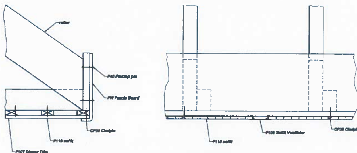
Figure 20bis – Mise en œuvre des lambris F110
