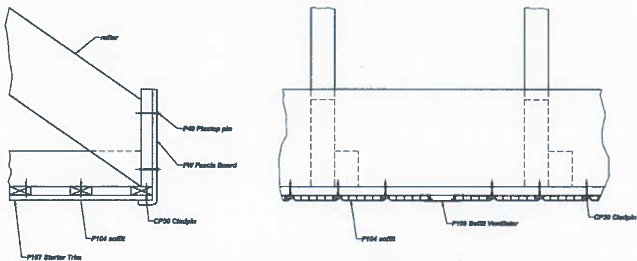
Figure 19bis – Mise en œuvre des lambris F104
