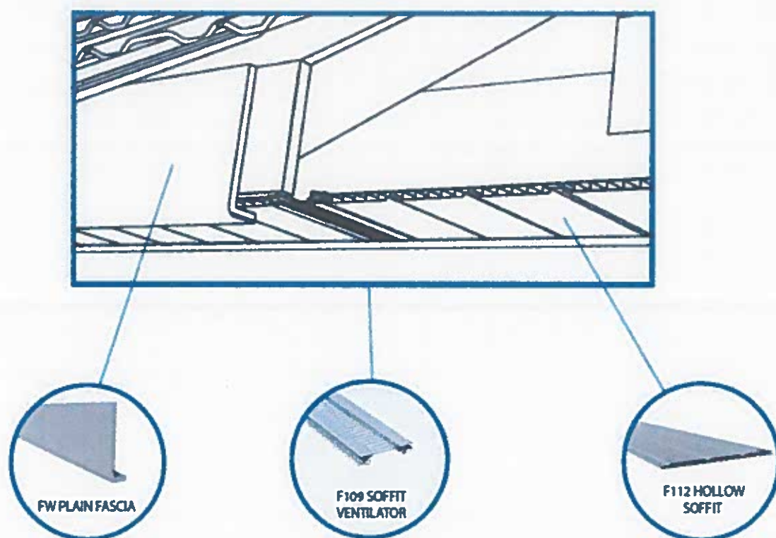
Figure 21 – Principe de mise en œuvre des lambris F112
