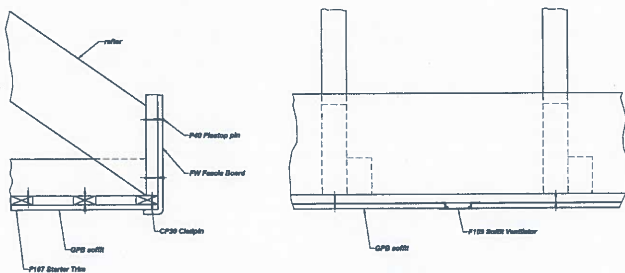
Figure 18bis – Mise en œuvre des planches GPB
