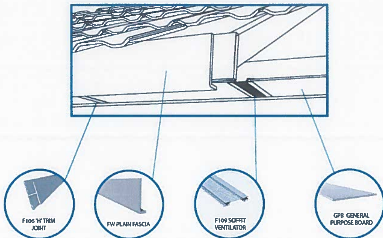
Figure 18 – Principe de mise en œuvre des planches GPB
