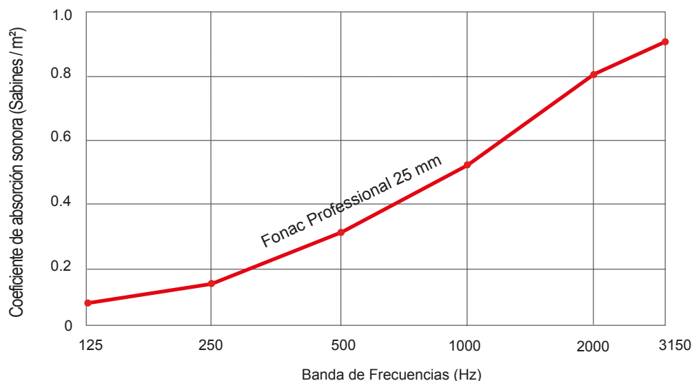
Curvas de atenuación sonora
