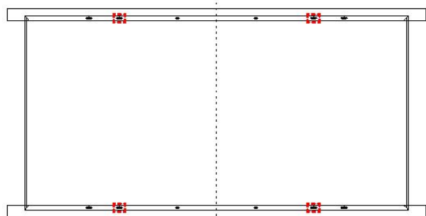
Instalación de 4 orificios internos sin viga transversal (B2)
