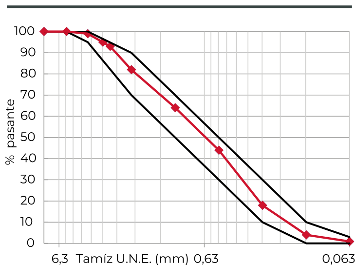
Curva granulométrica
