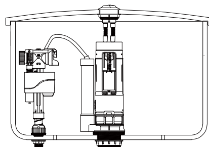
ENTRADA INFERIOR
