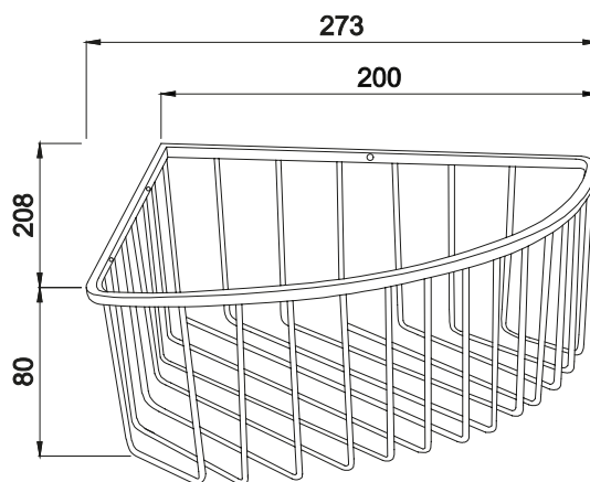
Esquema de dimensiones
