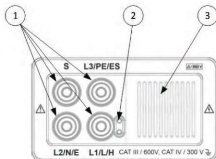
Figura 2.2: Panel de conexión
