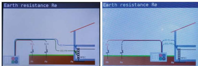
Figure 4.36: Diagrama de conexión a 4 hilos Figure 4.37: Diagrama de conexión a 3 hilos
