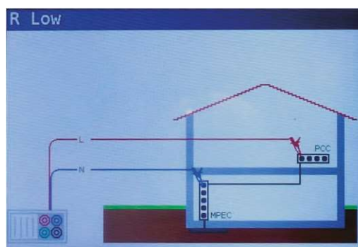
Figura 4 6: Conexión de los cables de prueba universales
