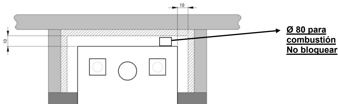
Imagen 3. Revestimiento del espacio de inserción – paredes combustibles y aislamiento
