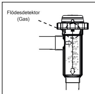
Fig. 5 REKOMMENDERAD installation
