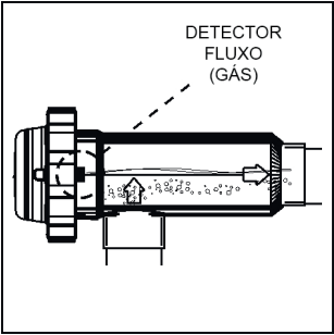
Fig. 6 Instalação PERMITIDA
