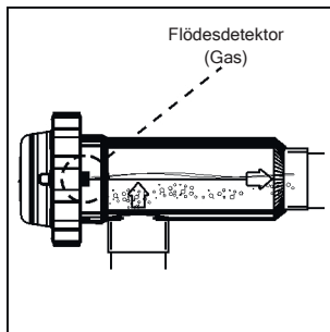
Fig. 6 GODTAGBAR installation
