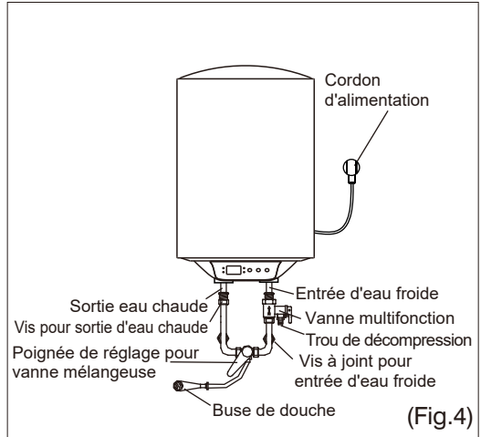
RACCORDEMENT TYPIQUE À PRISE UNIQUE
