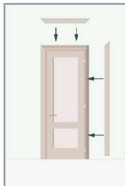
Figura 11. Fijación de Tapajuntas
