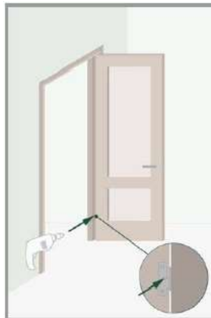
Figura 9. Fijación Definitiva del Cerco
