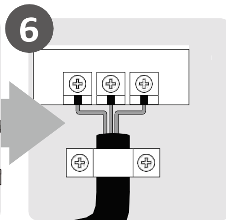
6 Conexión del cableado (pág. 19)
