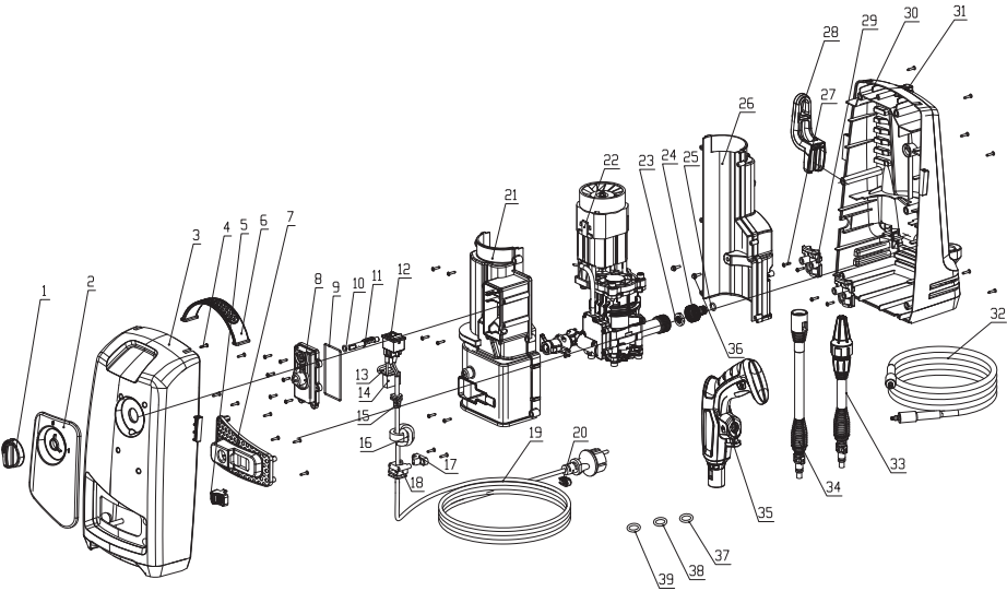
В) Зображення виробу в розібраному вигляді
