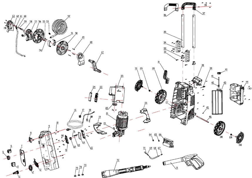
B) Produkt – widok rozstrzelony
