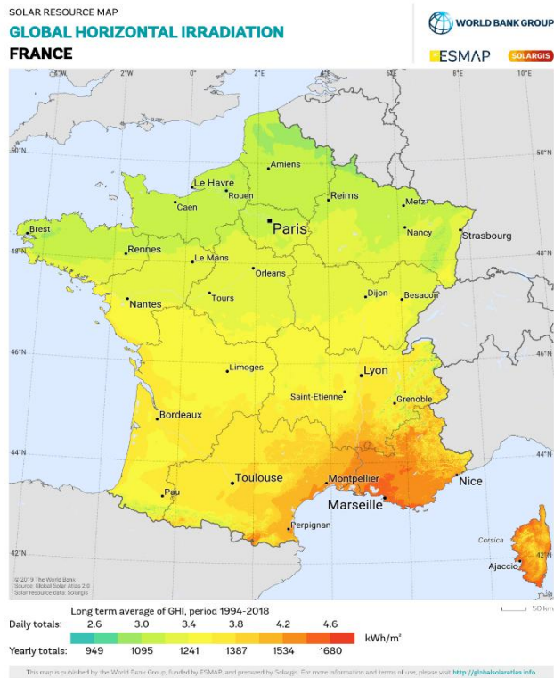
Figura 4 : Mapa de Francia de la irradiación horizontal global
