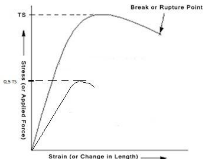
Figura 1: Resistencia a la tracción retenida tras la exposición a la radiación ultravioleta
