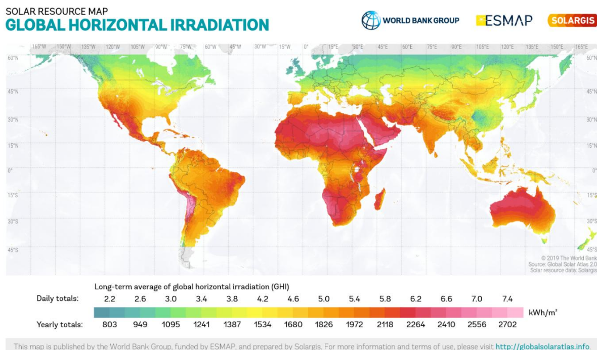
Figura 3 : Mapa mundial de la irradiación horizontal global
