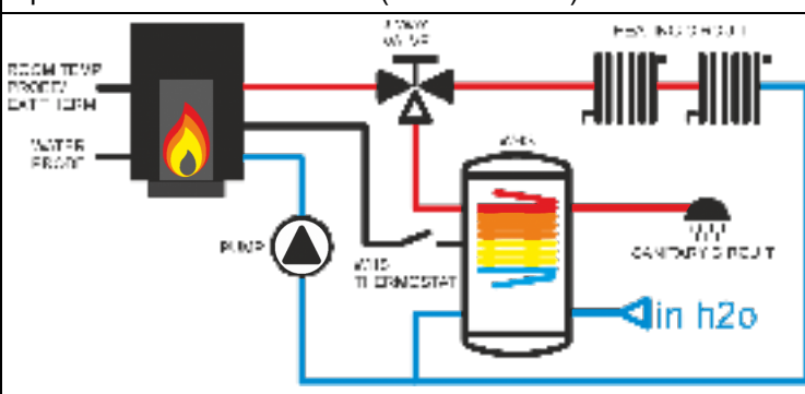
Tipo 4: caldeira de sonda (sem caldeiras)
