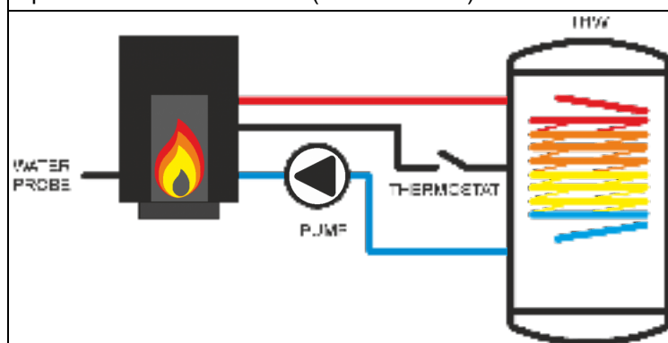
Tipo 5: buffer de sonda (sim caldeiras)
