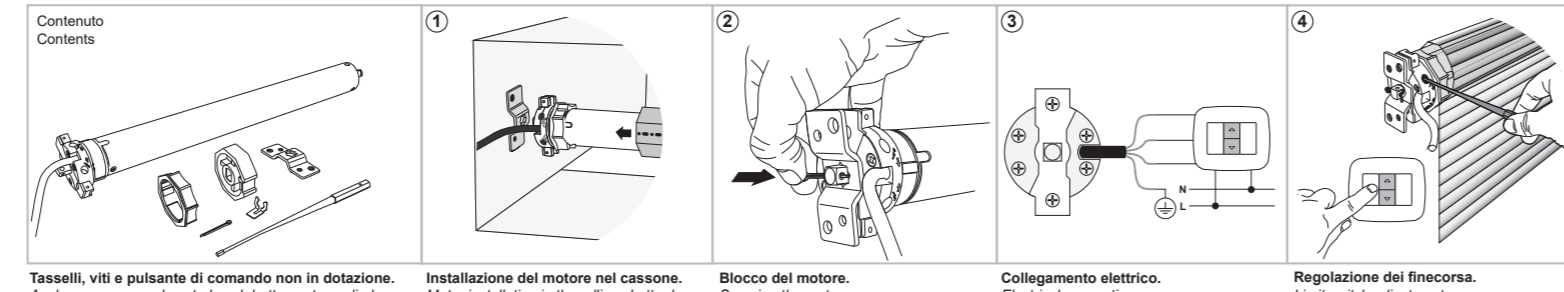
Tasselli, viti e pulsante di comando non in dotazione. Anchors, screws and control push button not supplied. Installazione del motore nel cassone. Motor installation in the rolling shutter box. Blocco del motore. Securing the motor. Collegamento elettrico. Electrical connection. Regolazione del finecorsa. Limit switch adjustment.
