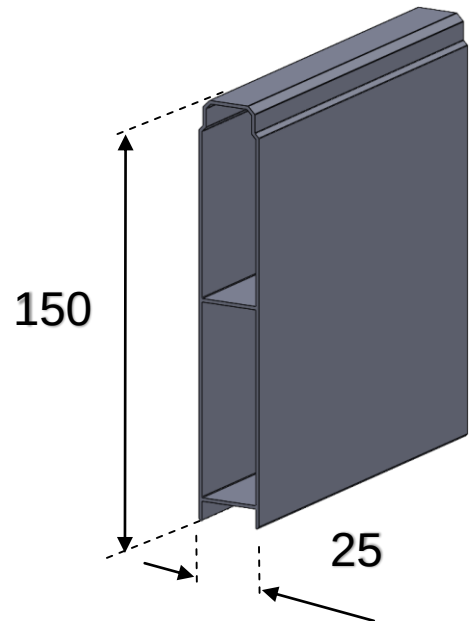
Lame pleine 150mm ép. 25mm
