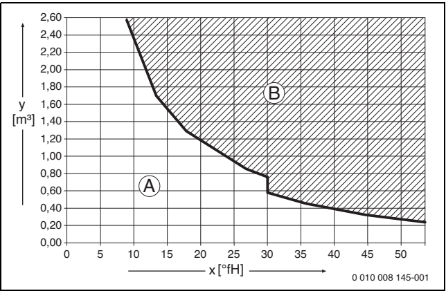
Fig. 18 Requisitos en aparatos <50 kW de agua de llenado y rellenado en °fH
