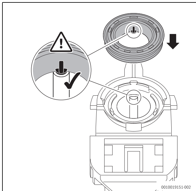
Fig. 49 Alinear la junta con el sifón de condensados
