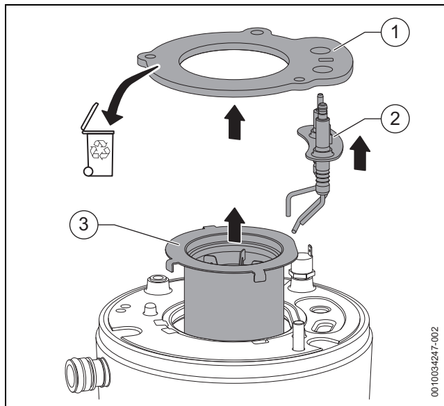
Fig. 41 Desmontar la cubierta del quemador
