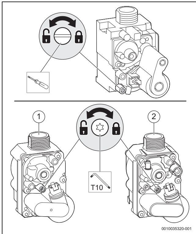
Fig. 33 Comprobar la presión de suministro de gas
