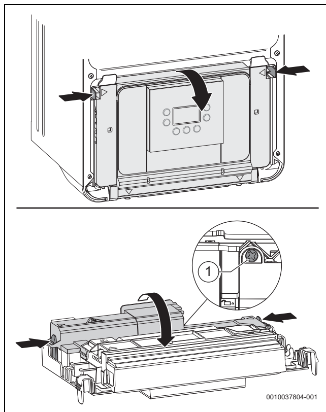
Fig. 25 Abatir la cubierta
