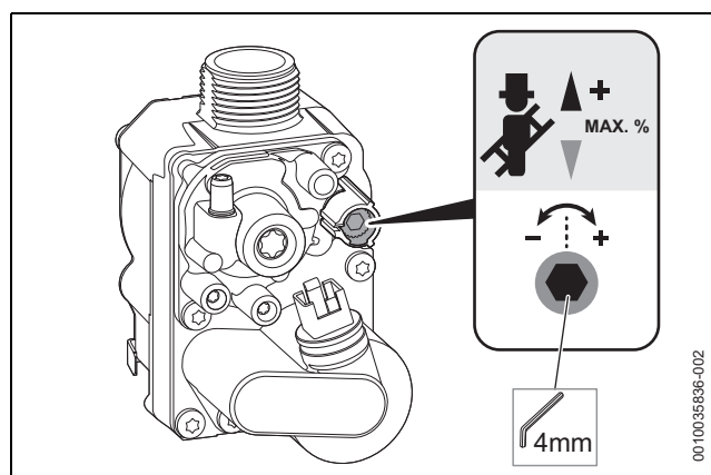
Fig. 36 Ajustar la concentración de CO 2 o de O 2
