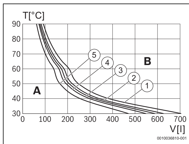
Fig. 19 Curvas para el vaso de expansión
