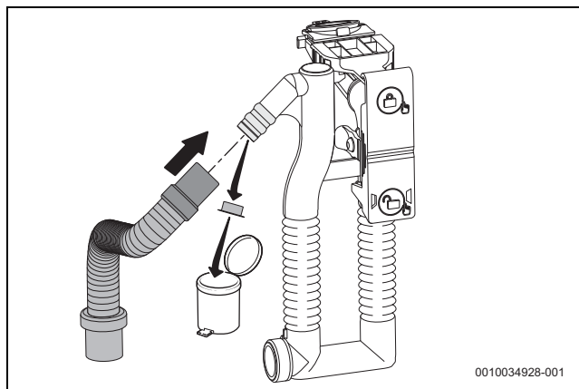
Fig. 22 Ajustar la manguera al sifón de condensado
