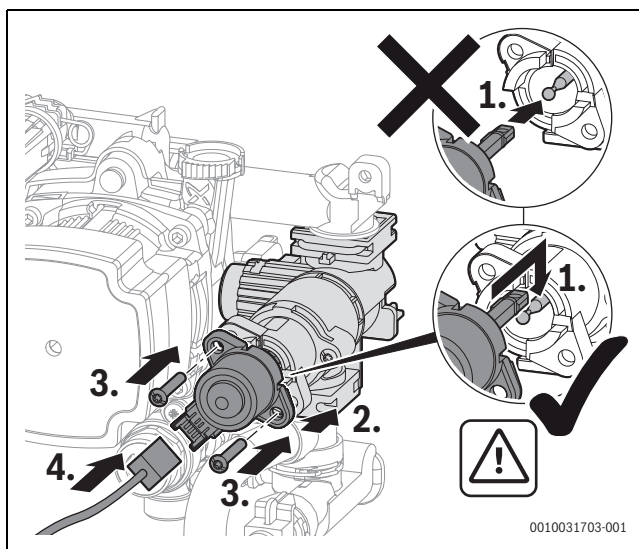
Fig. 60 Instalar el motor en la válvula de 3 vías (variante con tornillos)
