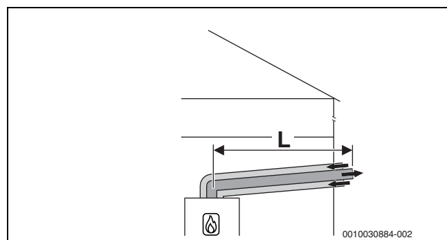
Fig. 8 Instalación de gas de evacuación concéntrica horizontal según C 13x a través de la pared externa
