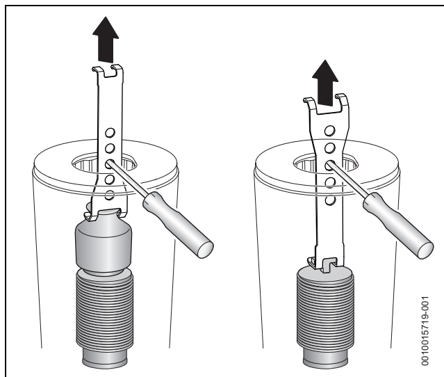
Fig. 42 Retirar la chapa guía superior e inferior
