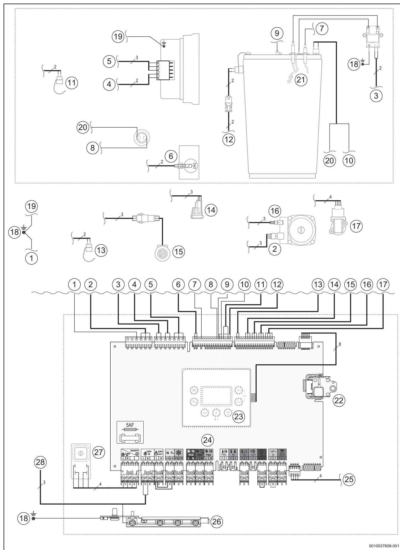
Fig. 66 Cableado eléctrico
