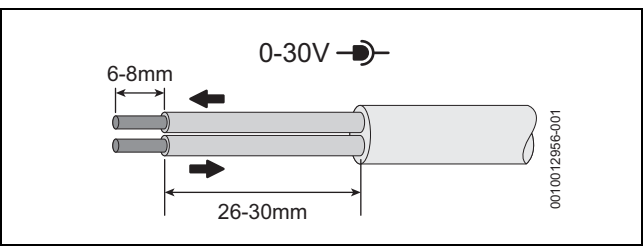
Fig. 28 Preparación de bajo voltaje (cables de señales)
