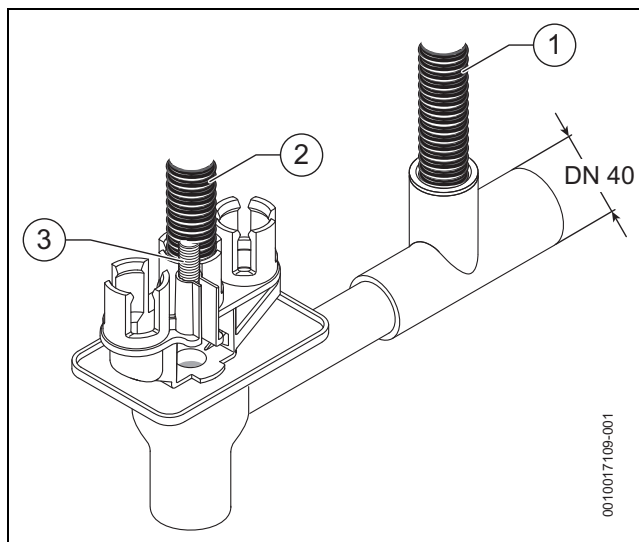
Fig. 23 Instalar los tubos de descarga en el accesorio de conexión 432
