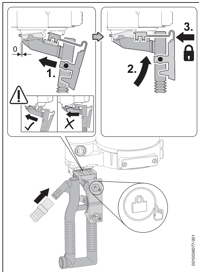
Fig. 51 Colocar el sifón de condensados
