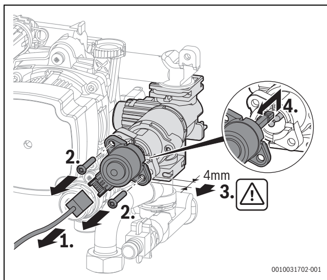
Fig. 59 Separar el motor de la válvula de 3 vías (variante con tornillos)
