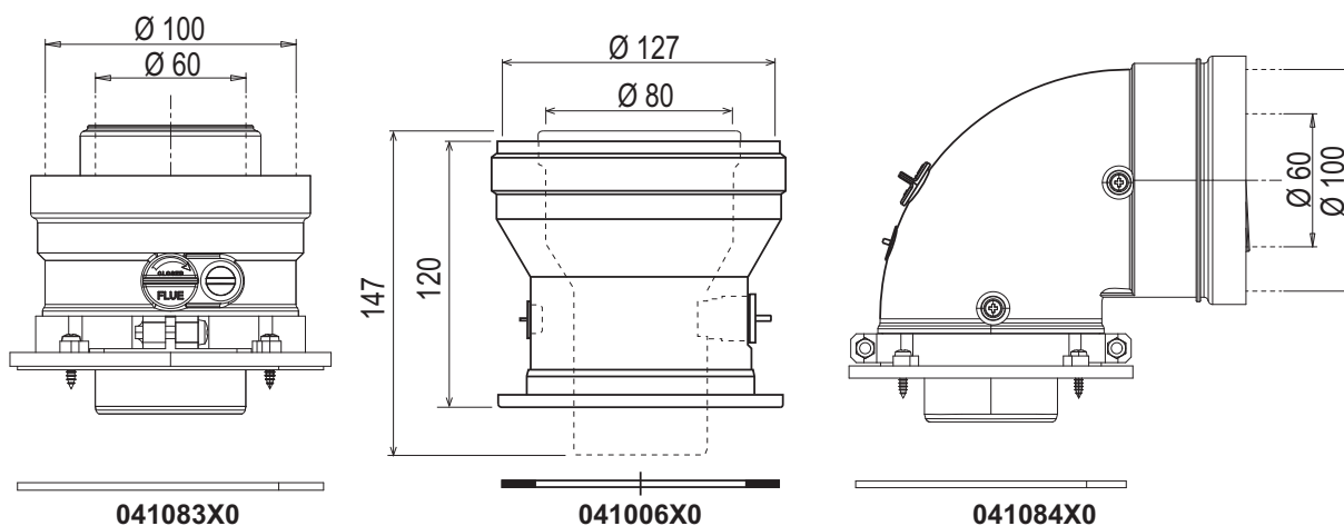
fig. 21- Accesorios iniciales para conductos coaxiales
