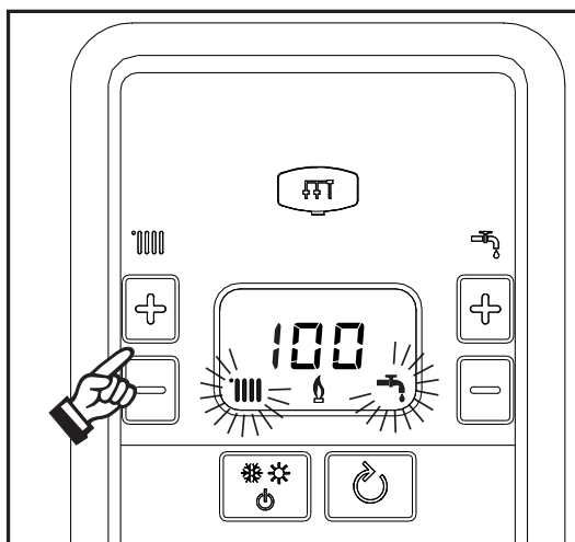
fig. 29- Modo TEST (potencia de calefacción = 100 %)
