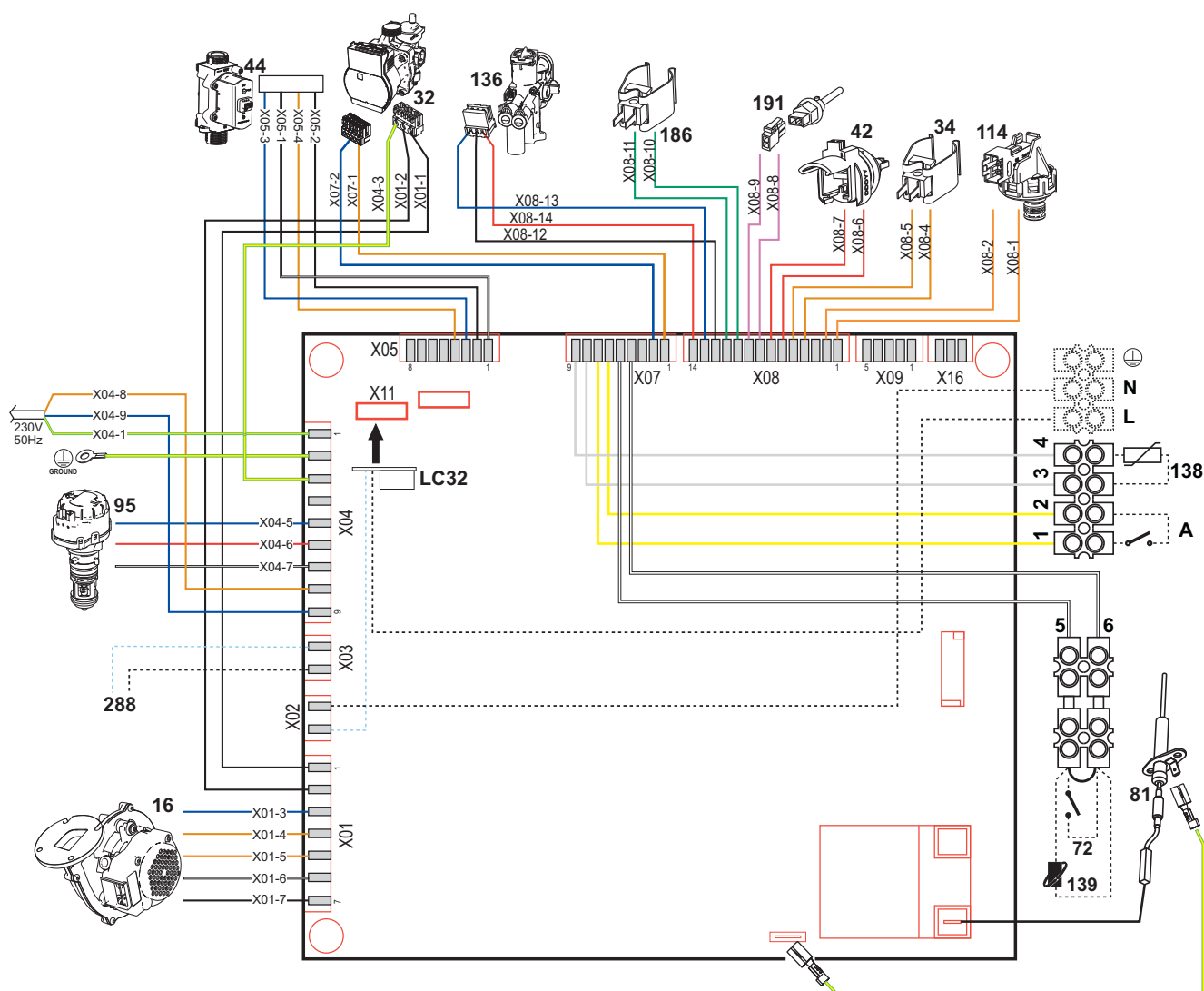
fig. 45- Esquema eléctrico
