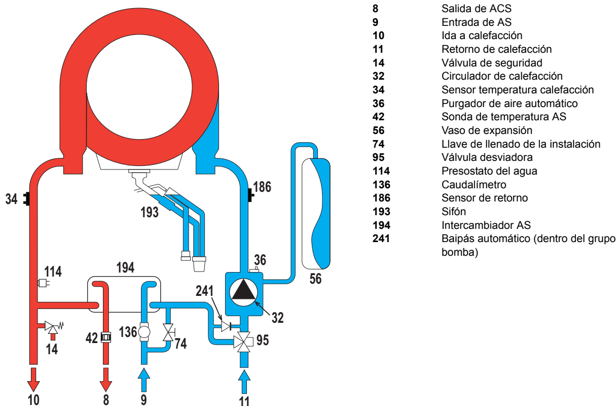
fig. 41- Circuito de agua
