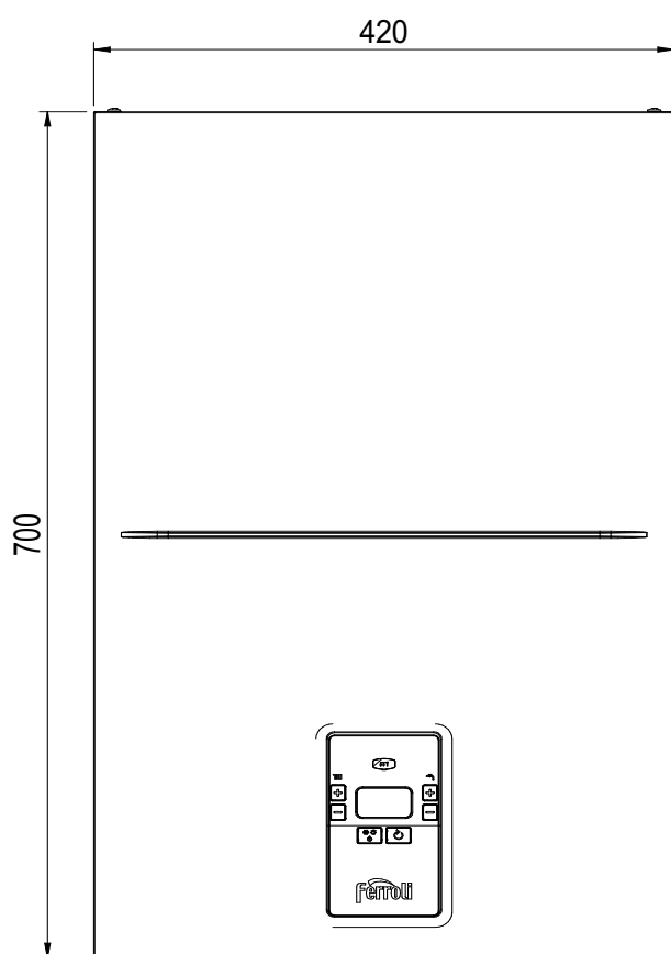
fig. 36- Vista frontal
