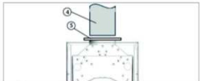
Figura 14 - Localização do dispositivo de segurança de exaustão de gases
