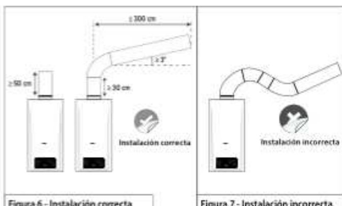
Figura 6 - Instalación correcta
