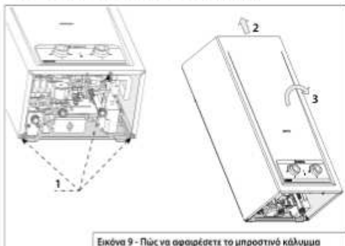
Εικόνα 9 - Πώς να αφαιρέσετε το μπροστινό κάλυμμα
