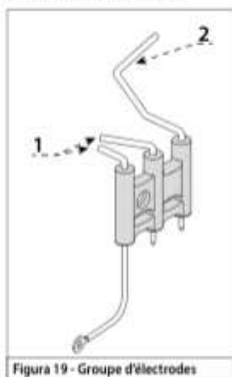
Figura 19 - Groupe d'électrodes
