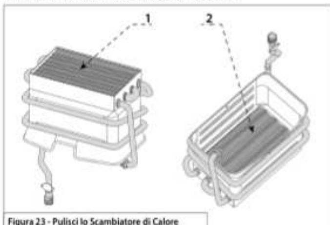
Figura 23 - Pulisci lo Scambiatore di Calore
