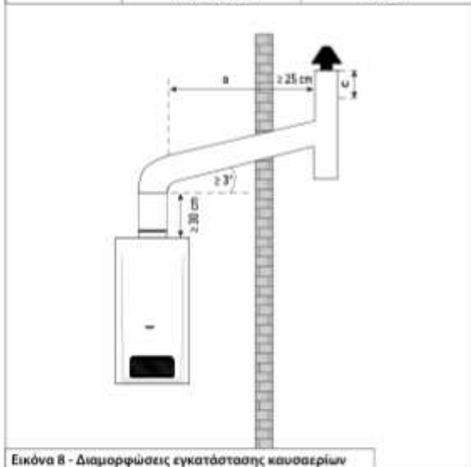
Εικόνα 8 - Διαμορφώσεις εγκατάστασης καυσαερίων
