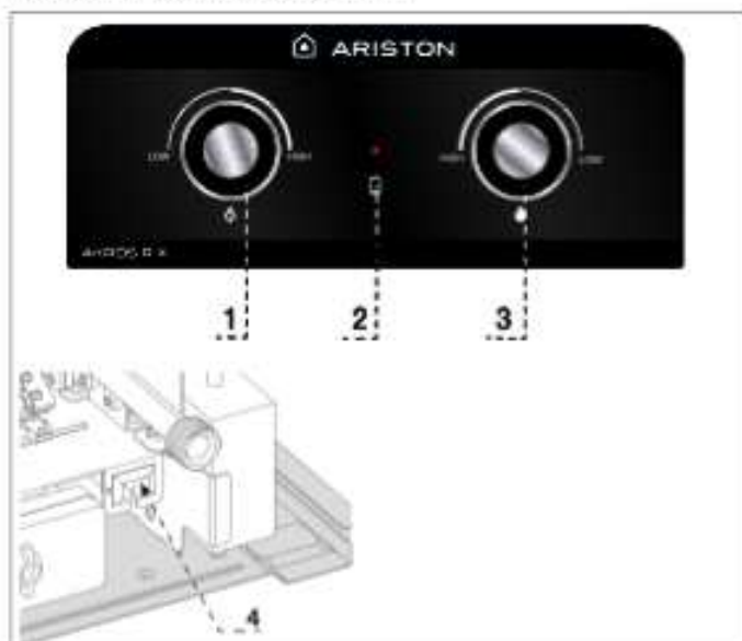
Figura 1 - Panneau de commande et bouton marche/arrêt
