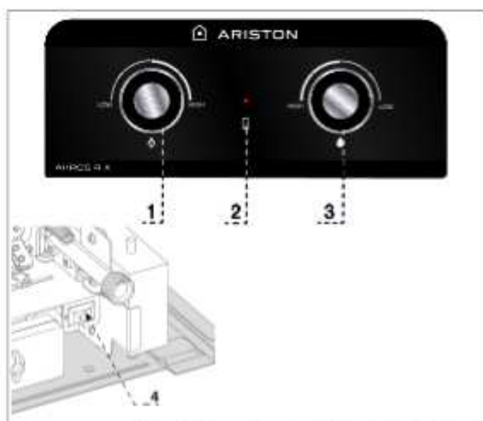
Figura 1 - Panou de control și buton Pornit/Oprit
