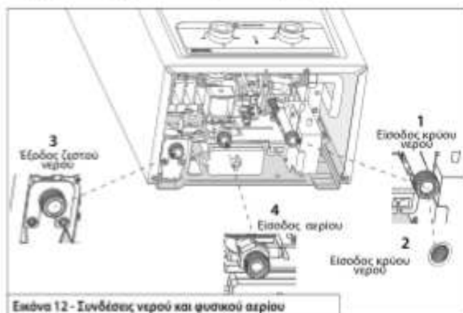
Εικόνα 12 - Σύνδεσεις νερού και φυσικού αερίου
