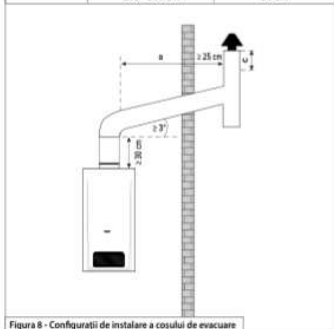
Figura 8 - Configurații de instalare a coșului de evacuare
