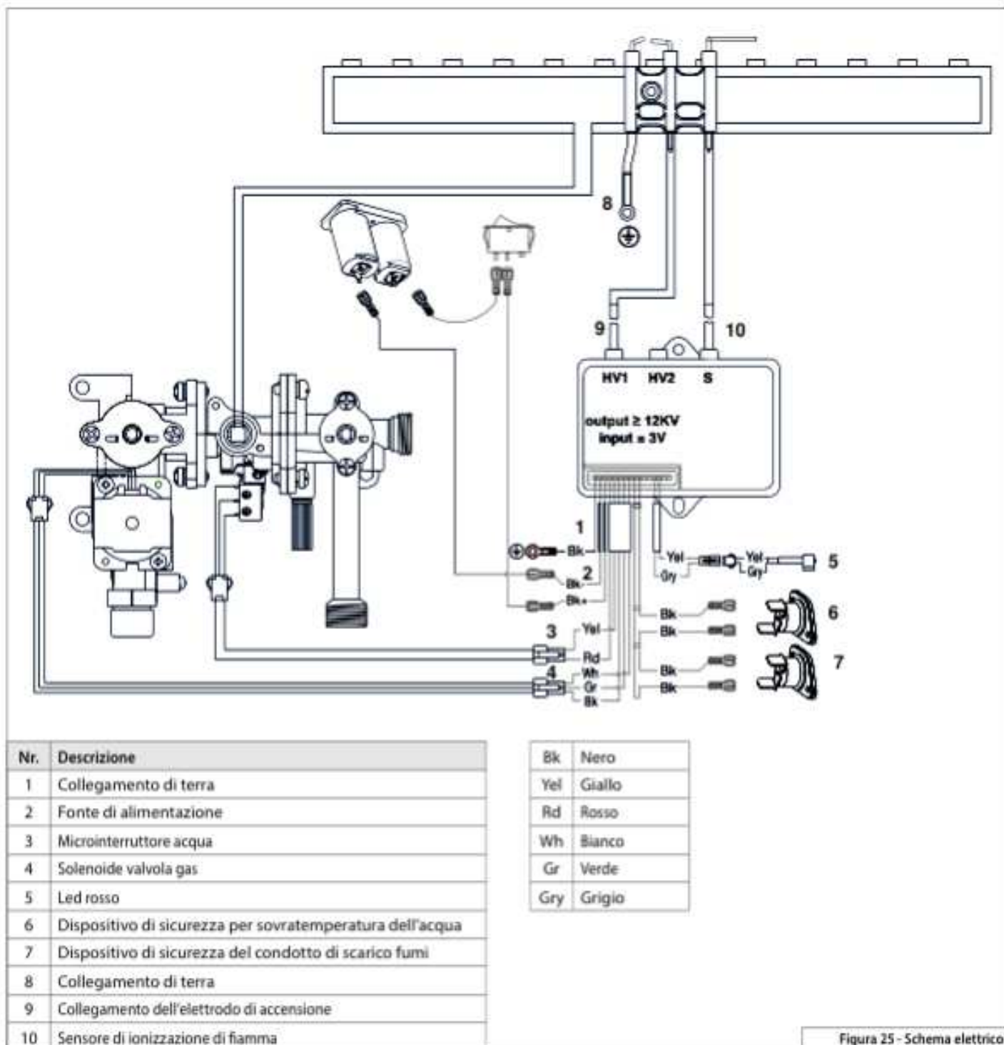
Figura 25 - Schema elettrico
