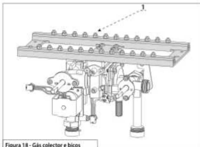
Figura 18 - Gás coletor e bicos
