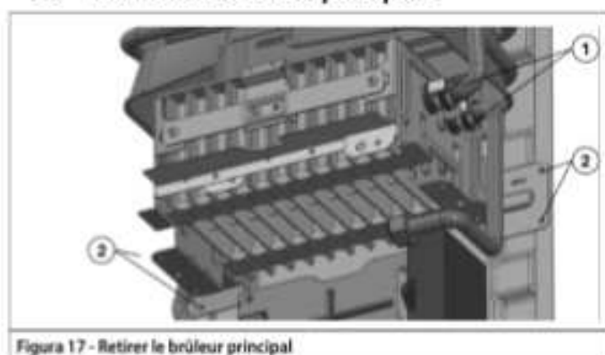
Figura 17 - Retrait du brûleur principal
