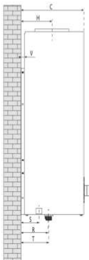
Figura 4 - Dimensiunile produsului
