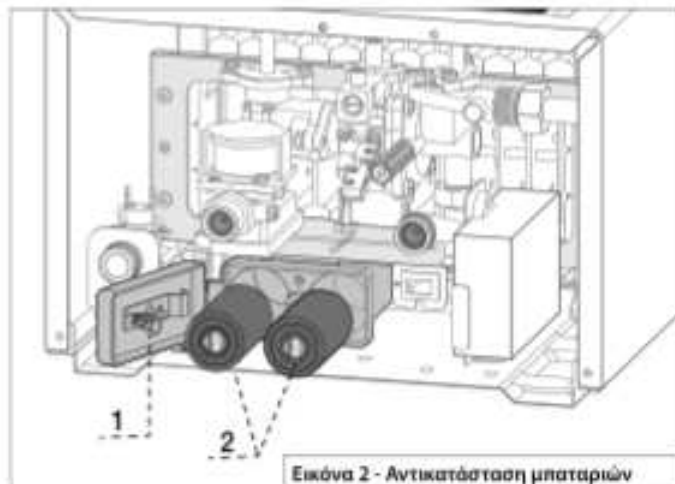
Εικόνα 2 - Αντικατάσταση μπαταριών
