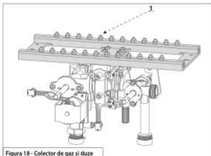
Figura 18 - Colector de gaz și duze
