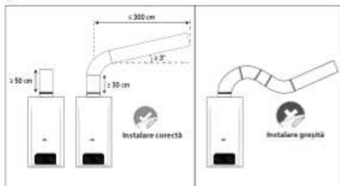
Figura 6 - Instalare corectă
