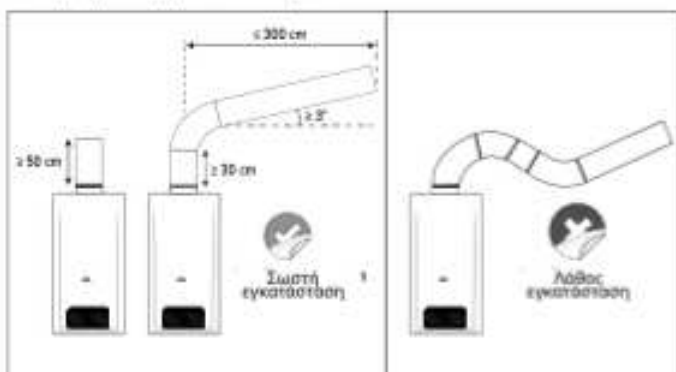
Εικόνα 6 - Σωστή εγκατάσταση
