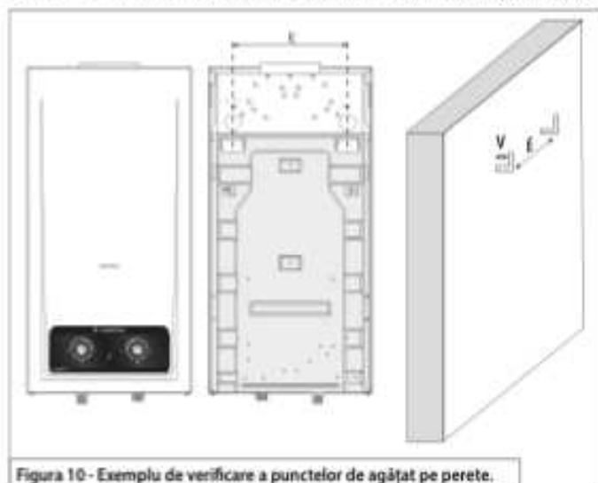
Figura 10 - Exemplu de verificare a punctelor de agățat pe perete.
