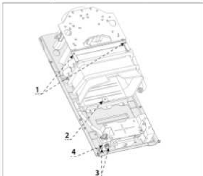
Figura 21 - Îndepărtați schimbătorul de căldură
