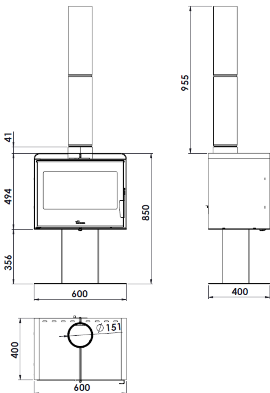
Figura nº1 - Dimensões em mm do aparelho Ocean/Atlantic 600
