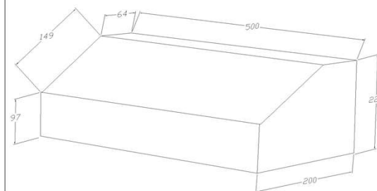
Bordillo 20x22x50
