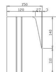
VISTA PERFIL
