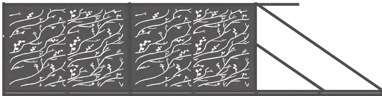
Brama przesuwna z zamkiem hakowym Szer. 4,00 m x Wys. 1,50 m L nr: 5905235218310 P nr: 5905235218327 Z automatem L nr: 5905235218334 P nr: 5905235218341
