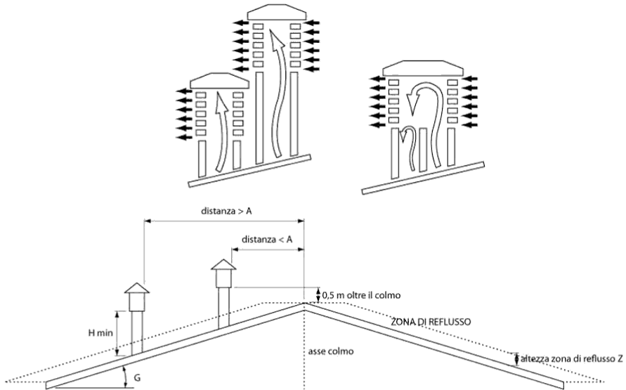
FIGURA 3.5/6 – Disposizione comignolo
