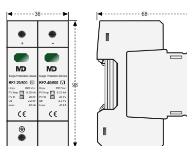
Dimensiones
