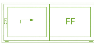
skrzydło przesuwne z boczną kwaterą nieotwieralną
