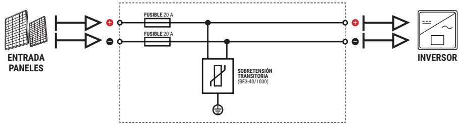
Esquema eléctrico SPF 1/1-40/1000/20 (226)
