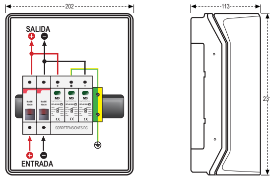
Plano de conexión SPF 1/1-40/1000/20 (226) y Dimensiones
