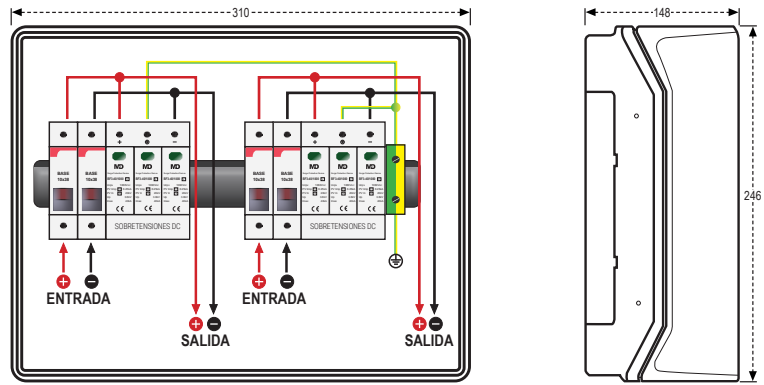
Plano de conexión SPF 2/2-40/1000/20 (226) y Dimensiones
