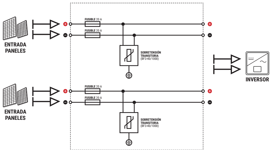
Esquema eléctrico SPF 2/2-40/1000/20 (226)
