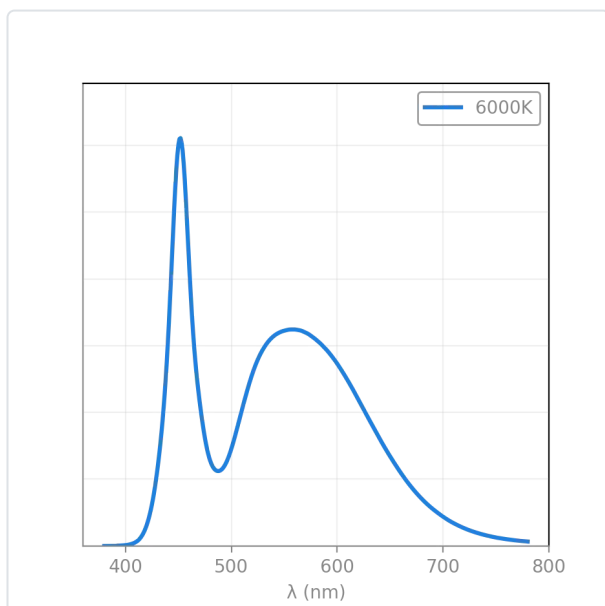
Distribuição espectral LPE2X25C60
