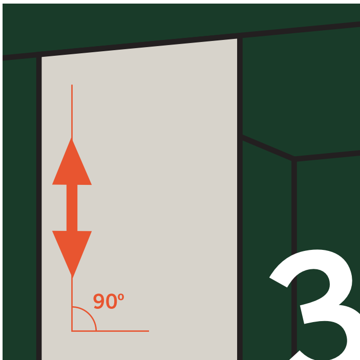
Fijación de la guía inferior: a. Comprobar, mediante el nivel, que la puerta quede vertical. b. Fijar la guía inferior con mastique o cinta adhesiva de doble cara si el suelo es de madera o radiante.
