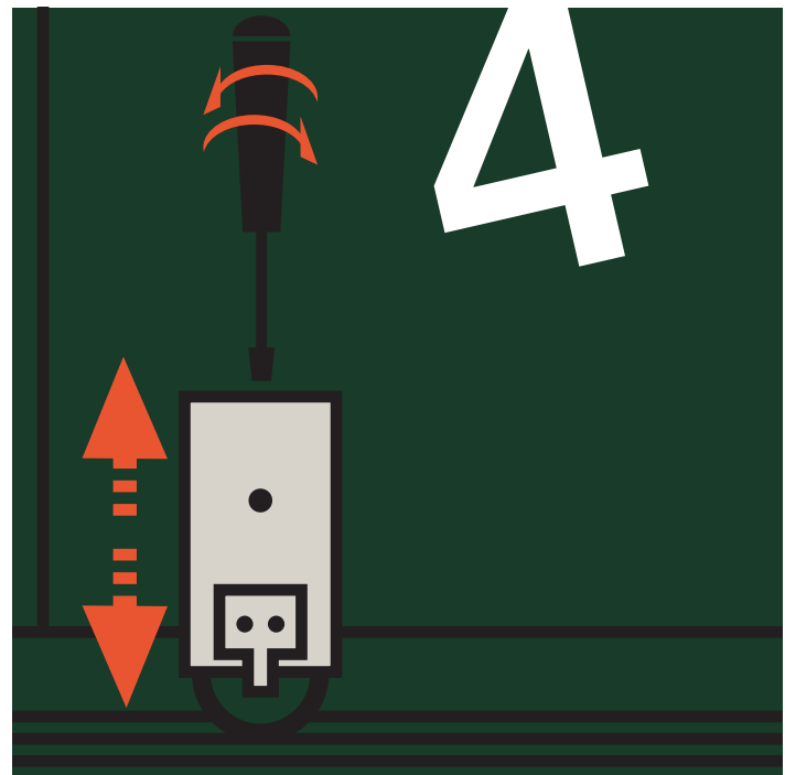
Ajustar la altura de las puertas con el destornillador, apretando o aflojando los tornillos de los soportes de las ruedas inferiores.
