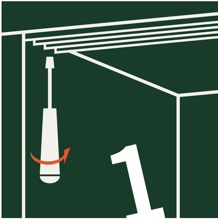
Fijar la guía superior atornillando los dos extremos.
