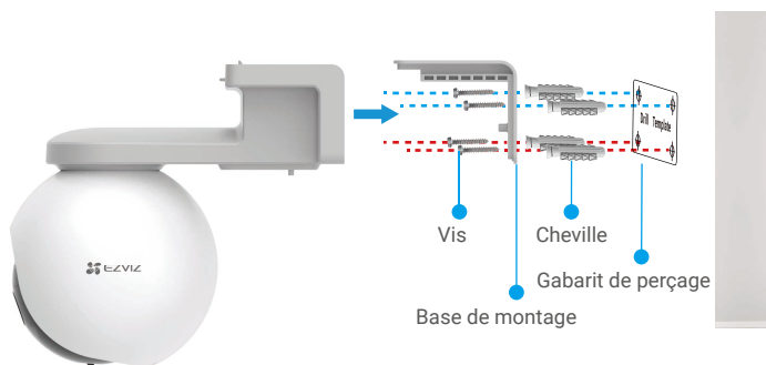
Fig. 2 Montage mural
