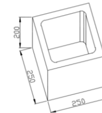
COLUMNA 250x250x200
