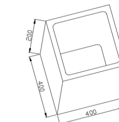
COLUMNA 400x400x200
