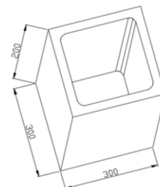
COLUMNA 300x300x200
