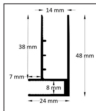
Profilé d'angle
