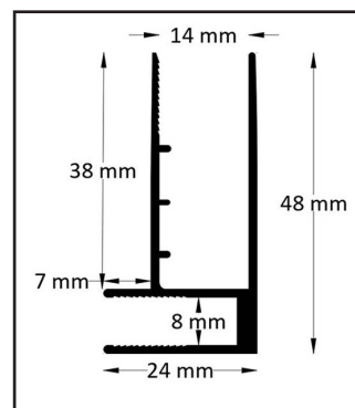
Profilo angolare
