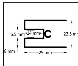
Profilé de verre fixe
