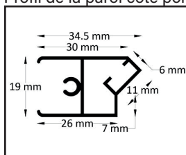
Profil de l'aimant
