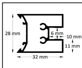
Profil de la charnière
