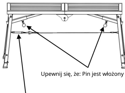
Wyreguluj napinacz
