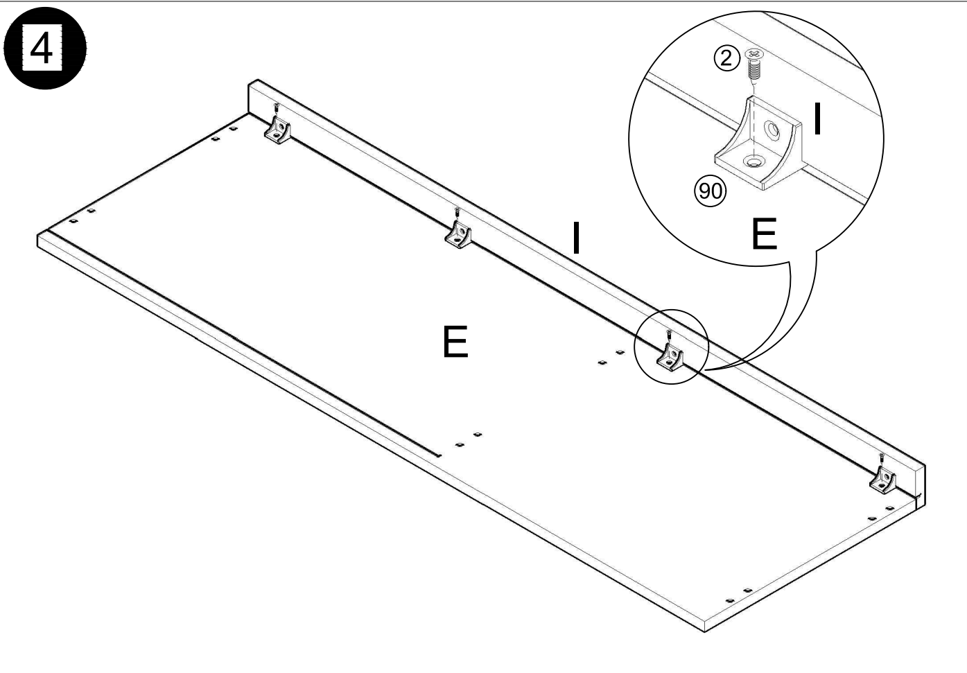
MÓDULO TV 1PTA.+HUECO 120x40 cm
