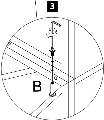
Assembler les 2 modules
