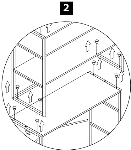
Retirer les caches des 2 modules au niveau de la jonction
