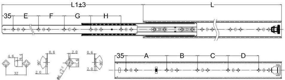
Patrón de orificios de instalación 5301/5301Z (Unidades: mm)
