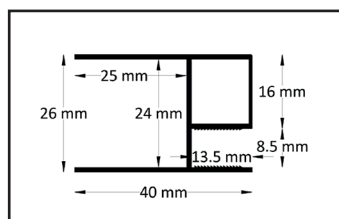
Profil de maintien du verre fixe
