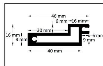
Barre de roulement des roues
