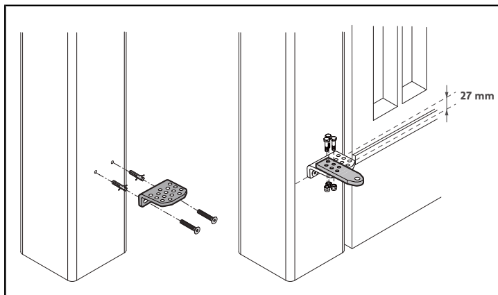
Patte à visser
