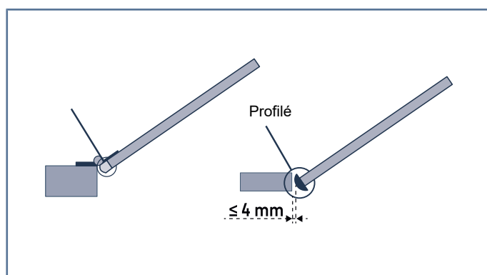
Fig. 2: Protection mécanique
