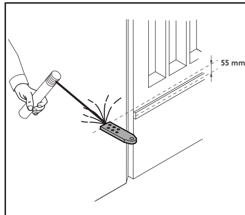
Patte à souder
