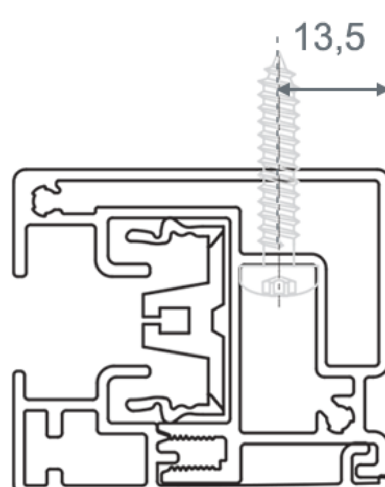
Pose de face
