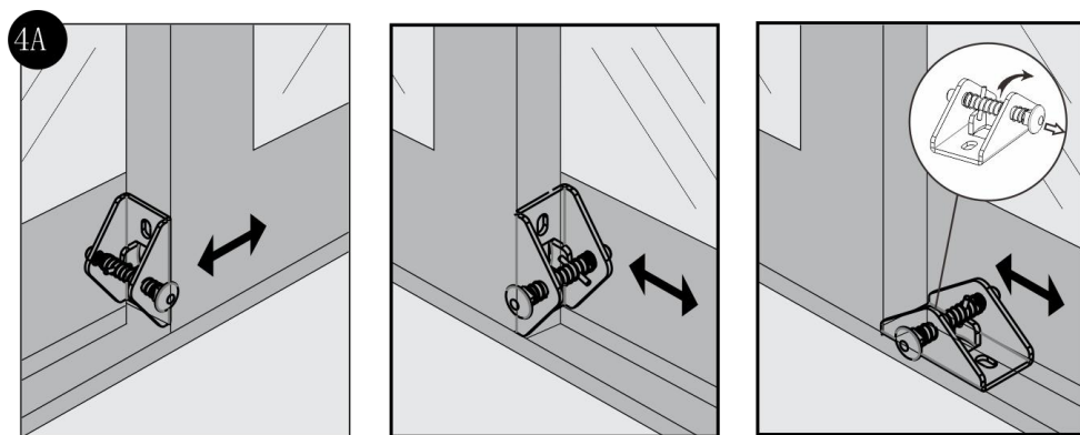
Grendelmontage op schuifdeur
